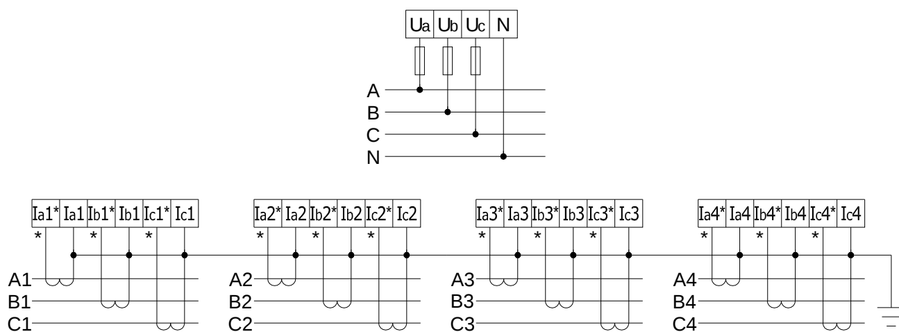
三相四线
